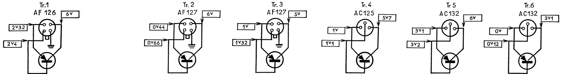
TENSIONS MESURÉES AVEC VOLTMETRE A LAMPE EN PO EN L'ABSENCE DE SIGNAL
