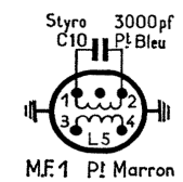
SCHEMA REPRESENTÉ COMMUTÉ EN PO
