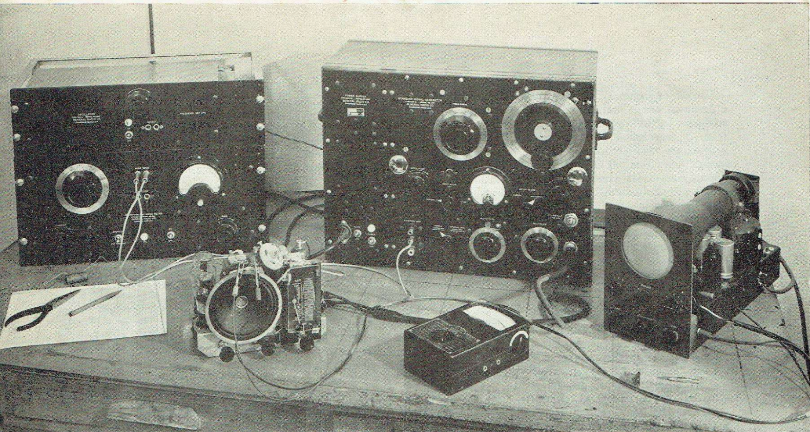
Mesures du coefficient de distortion non linéaire, au cours de l'essai du récepteur Intégra type S.B.5. A gauche, le générateur à 800 périodes de la General Radio, donnant une onde sinusoïdale pure ; à la partie inférieure, on trouve le pont de mesure du taux de distortion qui donne ce taux en lecture directe. Au milieu, le générateur General Radio 605 A qui a servi à relever les caractéristiques du récepteur. La mesure des tensions de sortie se fait au moyen d'un voltmètre à redresseur, contrôlé lui-même par un oscillographe cathodique (Brillon-Leroux et Compagnie des Compteurs). Au premier plan, le récepteur en étude ; on remarque au-dessus du haut-parleur un réostat dont la résistance a été ajustée à une valeur égale à l'impédance motionnelle de la bobine mobile à 800 périodes.
