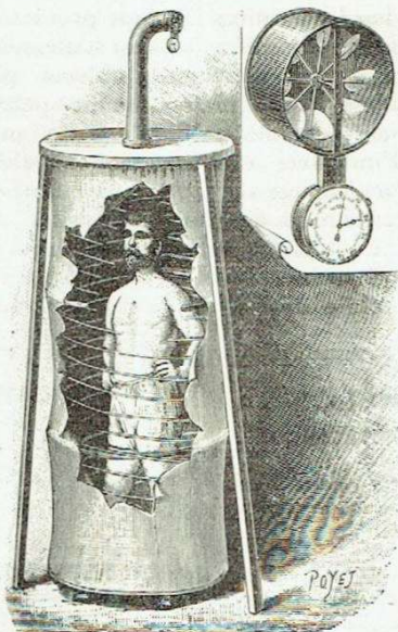
Fig. 1. — Extrait de la « Revue Générale des Sciences » du 15 mai 1894, p. 322. Expérience de calorimétrie : le sujet se tient debout, dans l'axe d'un solénoïde parcouru par un courant de haute fréquence. Une enveloppe de laine forme l'enceinte calorimétrique. On peut ainsi mesurer l'effet vasodilatateur des courants radioélectriques.
