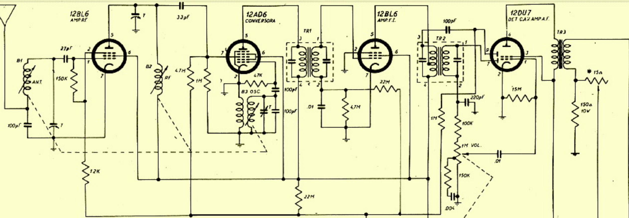
Autoradio Peugeot 403 modelo 460 P
