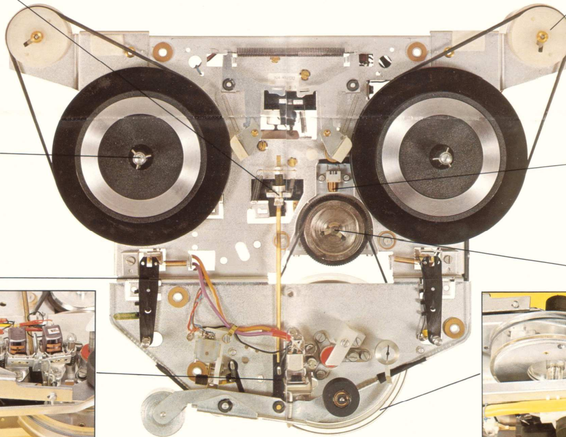
N 4418 Die Betätigung der Andruckrolle und Kopf- abschirmungen erfolgt elektromagnetisch.
