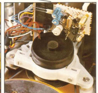
N 4414 Tachogeregelter Capstan-Motor mit Ansteuerungselektronik (Rückseite).
