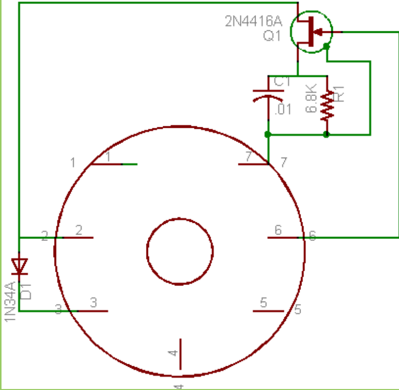
1L4 Module RT77/GRC-9 V1 RF Amplifier
