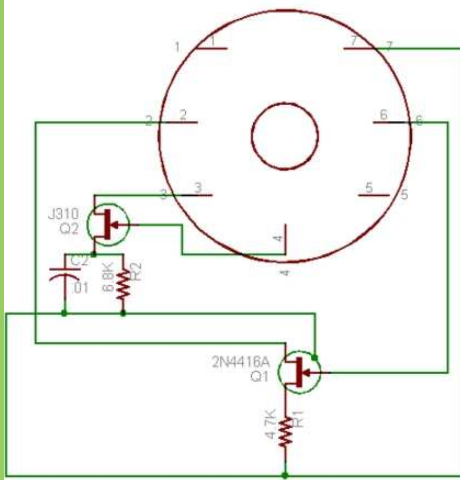
1S5 Module RT77/GRC-9 V5 Det/AVC/Preamp
