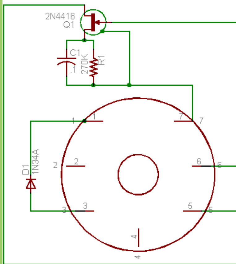
1S5 Module RT77/GRC-9 V5 Det/AVC/Preamp
