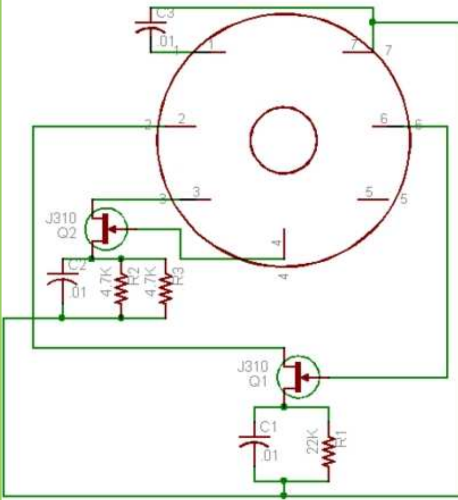
1L4 Module RT77/GRC-9 V3 I.F. Amplifier
