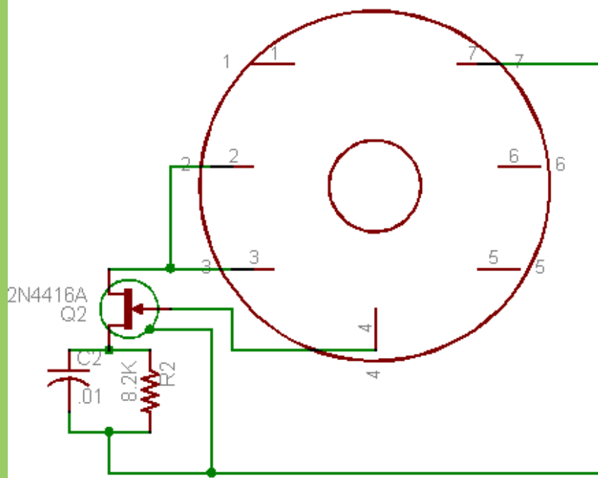
1R5 Module RT77/GRC-9 V7 BFO Oscillator
