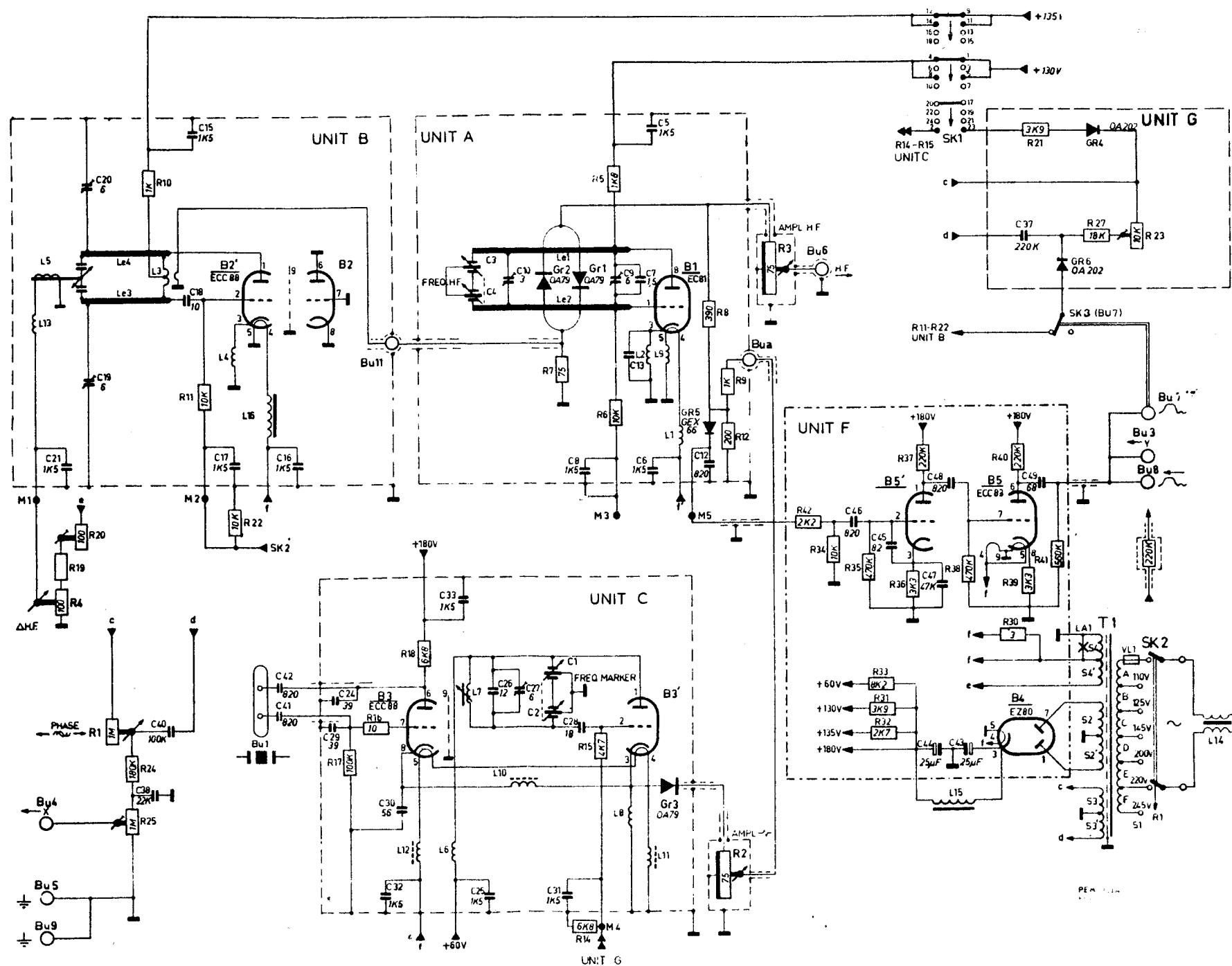
Fig. 25. Circuit diagram
