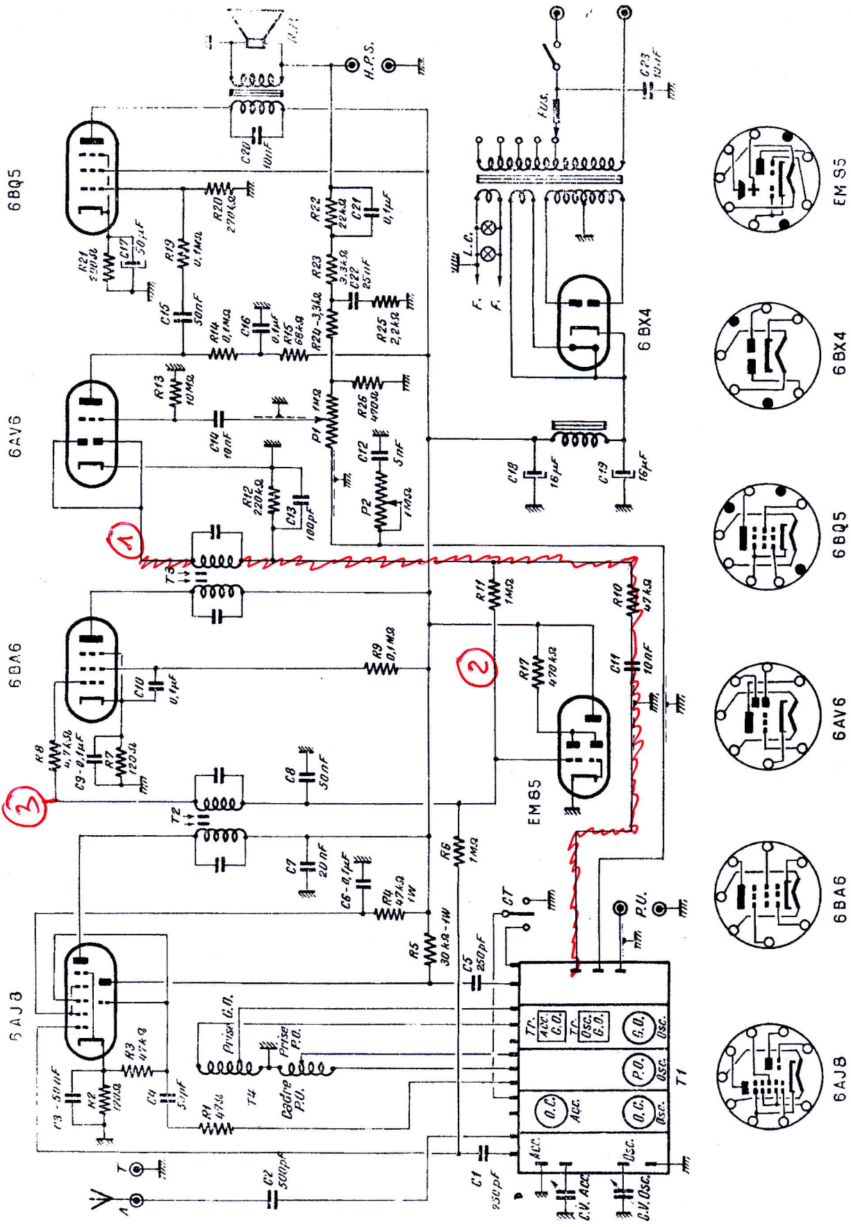
Schéma général du récepteur 5726. Voir également d'autres détails à la page 30.
