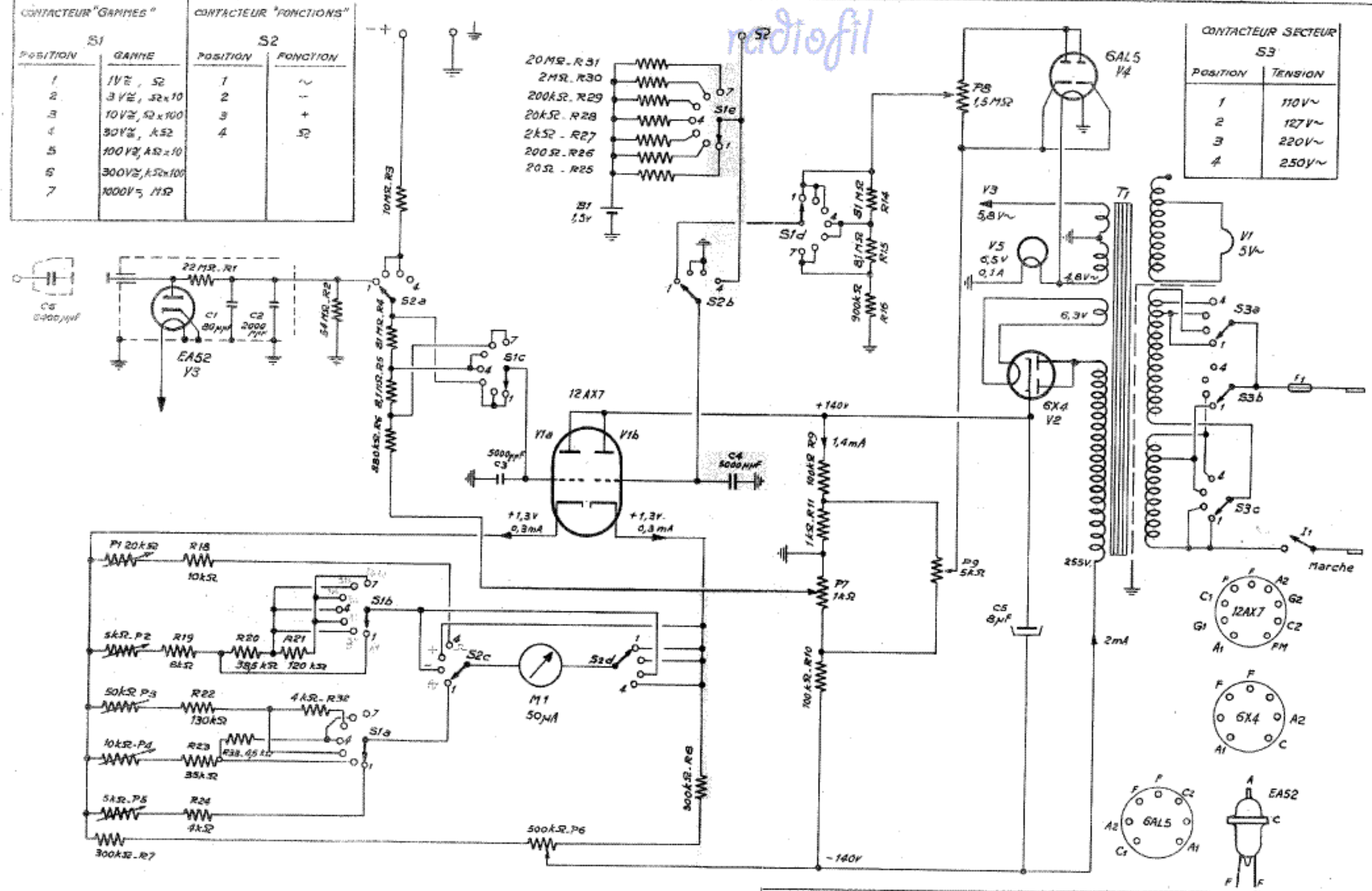
VOLTOHMMÈTRE ÉLECTRONIQUE-744-METRIX SCHEMA DE PRINCIPE
